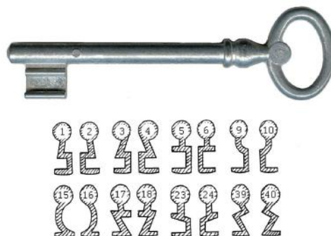
7. ábra KERTKAPU HAJLÍTOTT Profil
