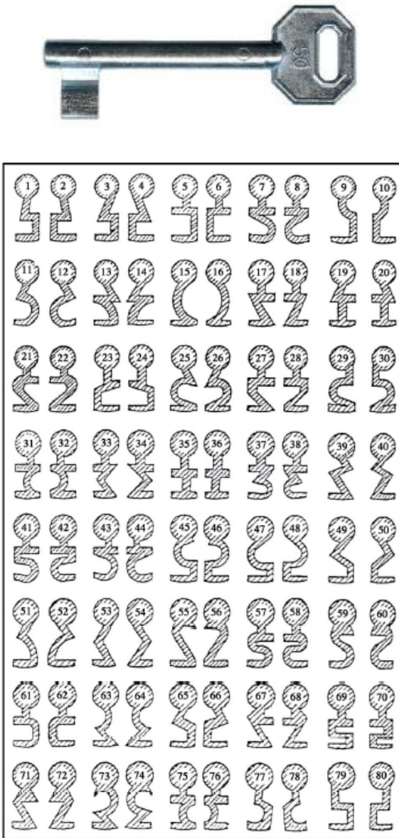
4. ábra SOPRONI RÉGI HAJLÍTOTT Profil, Lővér zárakhoz
